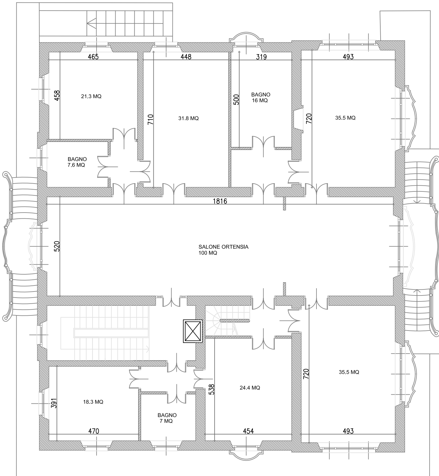
PIANTA PIANO SUPERIORE
